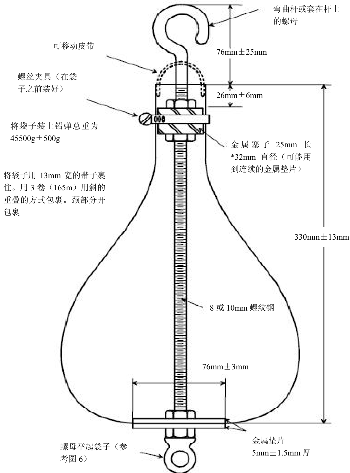
图 4 撞击袋
